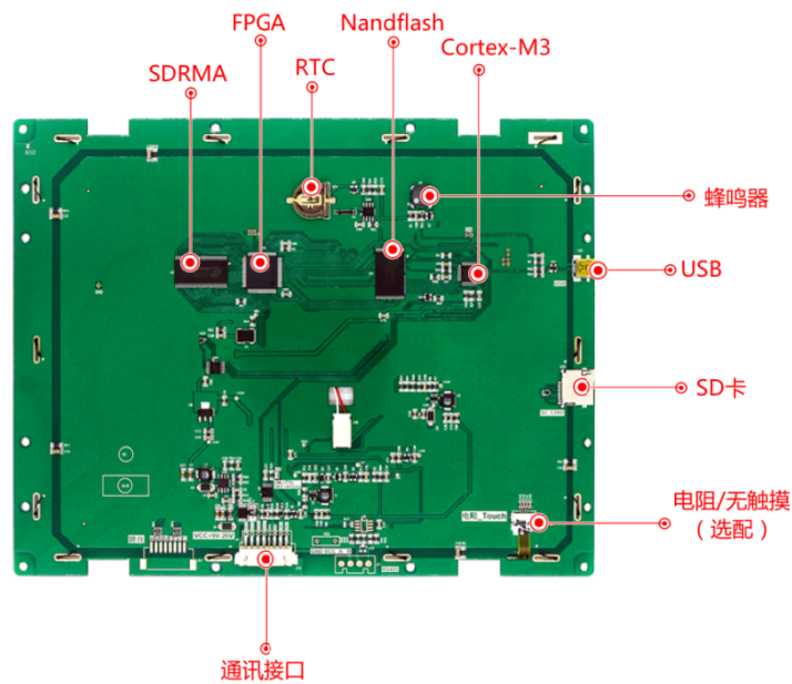
图 1-3 硬件配置图
