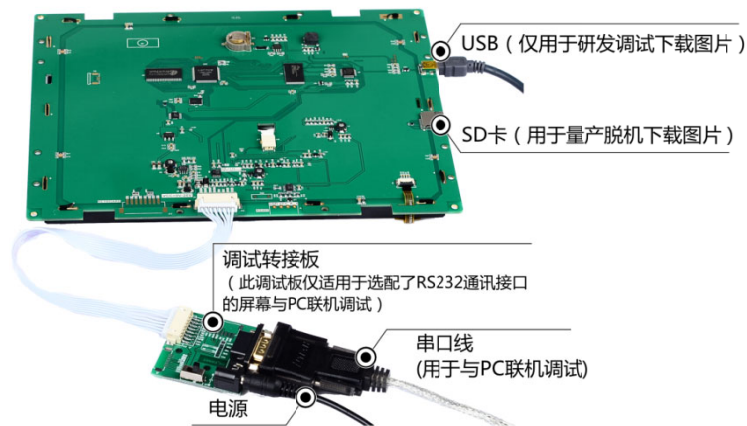
图 1-4 调试工具图
